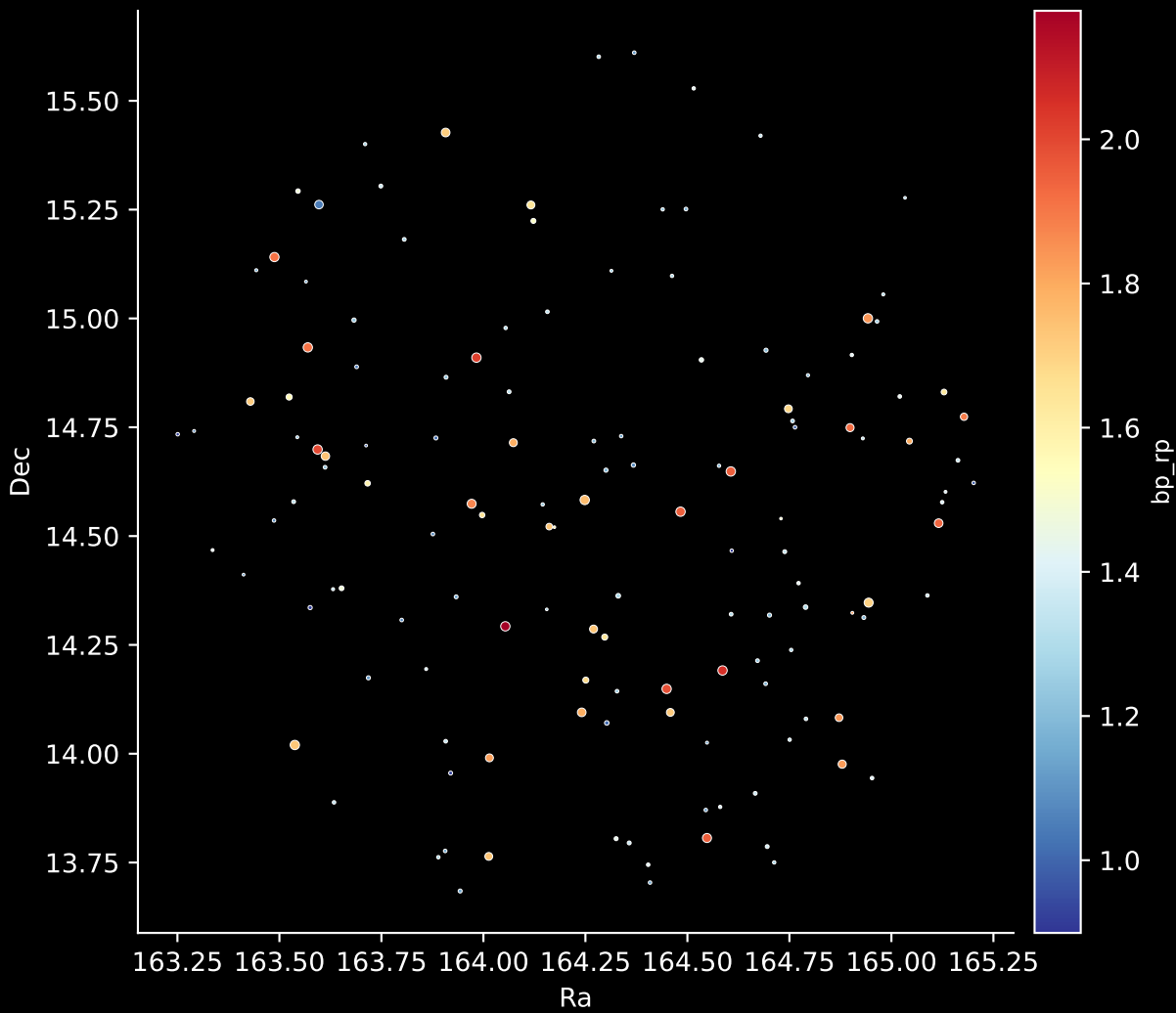
GALAH DR4 Field: [6586] Stars: 137
