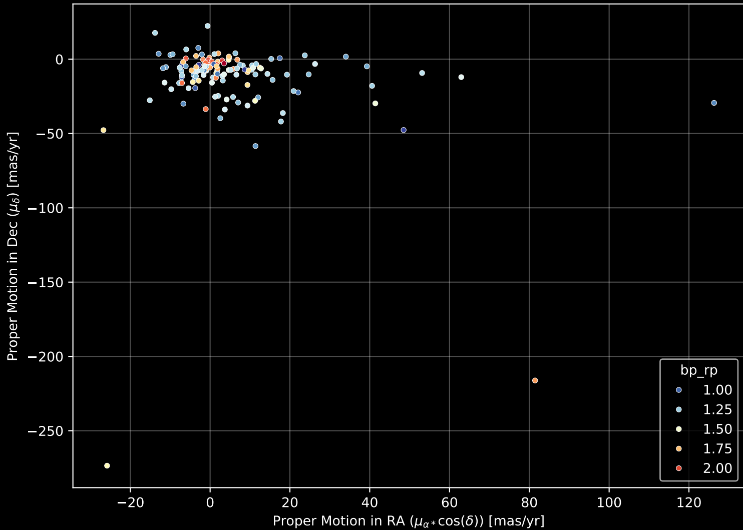
GALAH DR4 Field: [6586] Proper Motion Diagram (n= 137)
