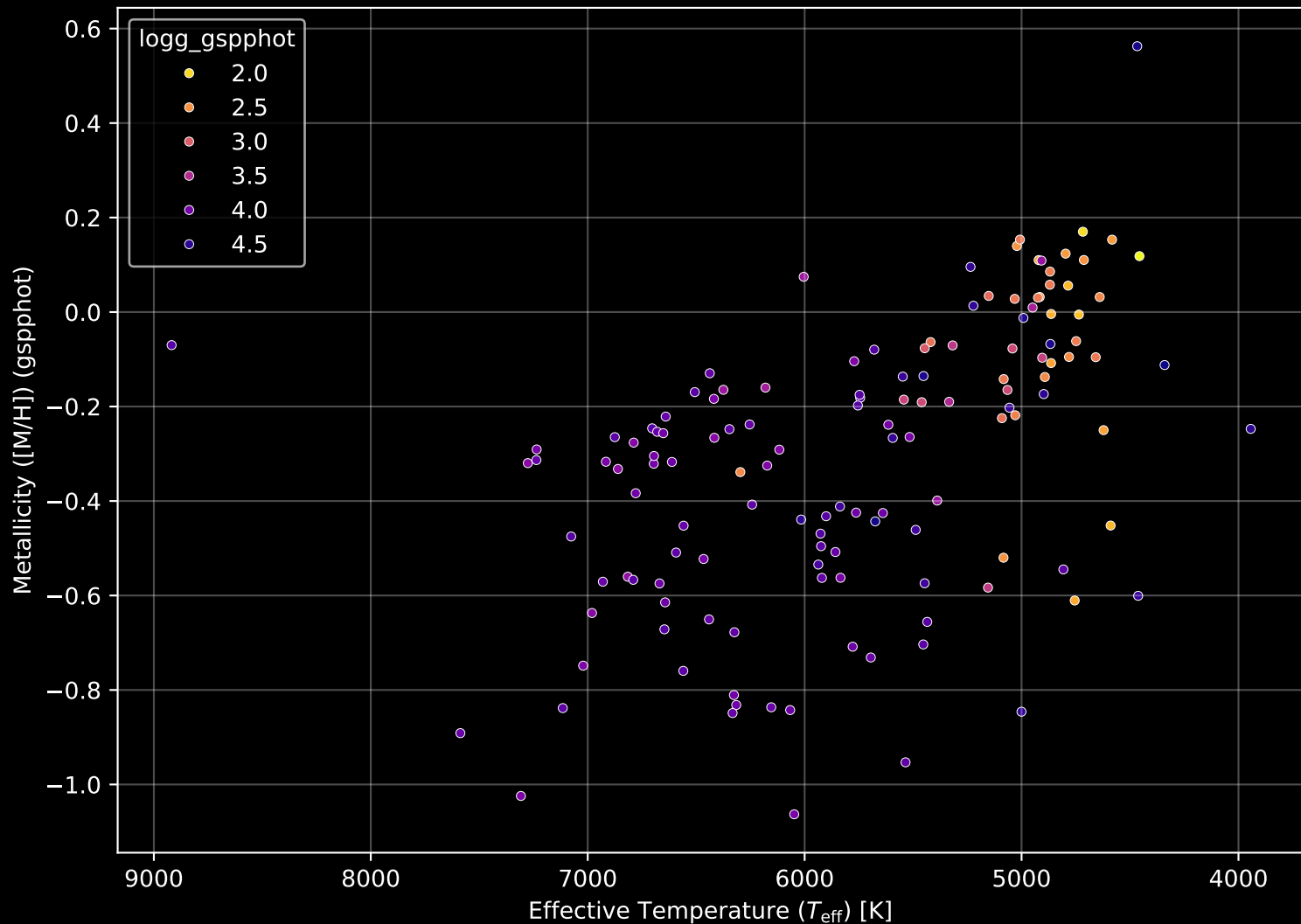
GALAH DR4 Field: [6586] Stellar Population Parameters (n= 137)
