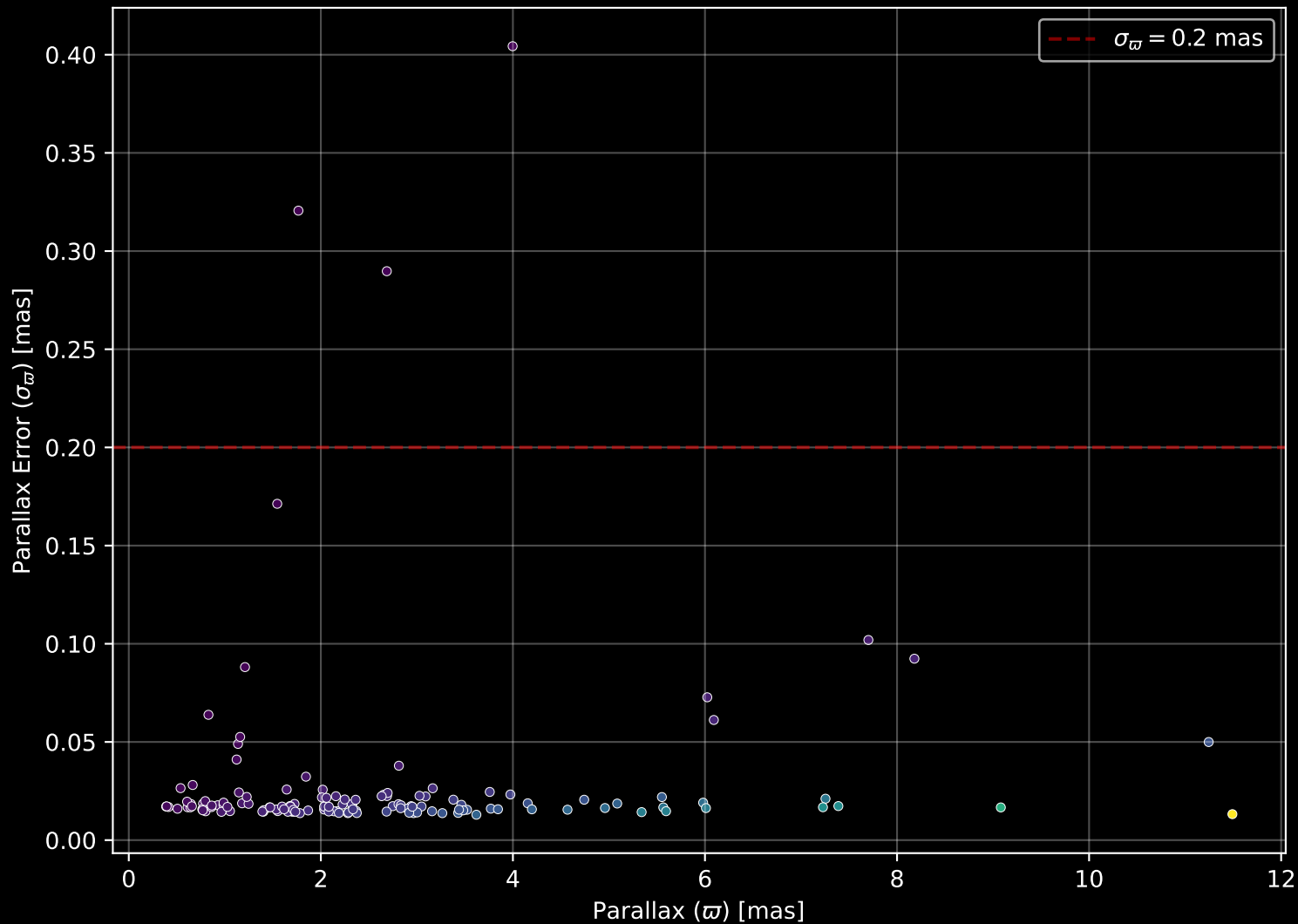
GALAH DR4 Field: [6586] Parallax Quality (n= 137)
