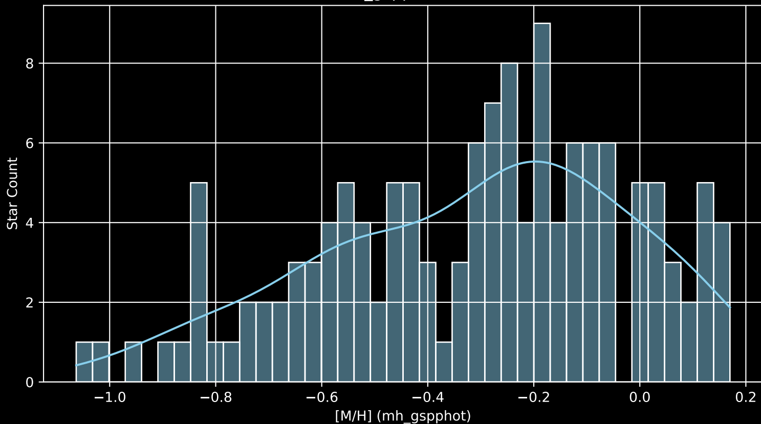
GALAH DR4 Field: [6586] [M/H] (mh_gspphot) (n= 136)
